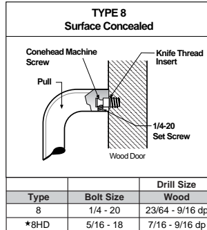
Wood Door - Type 8
