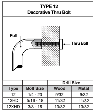
Wood or Metal Door - Type 12
