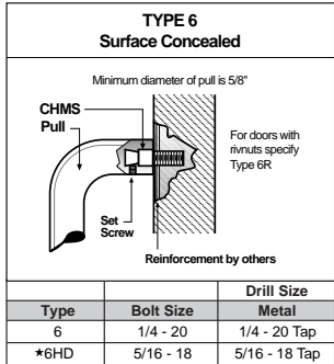
Metal Door - Type 6
