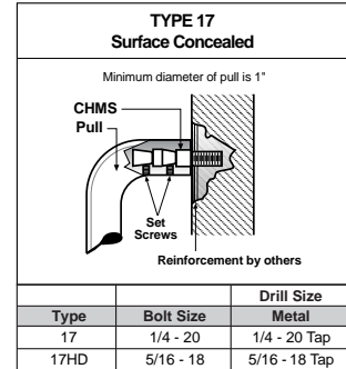
Metal Door - Type 17
