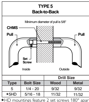
Wood or Metal Door - Type 5
