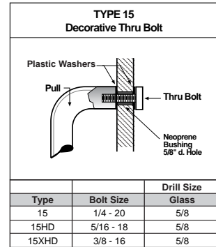
Glass Door - Type 15
