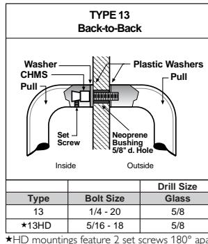
Glass Door - Type 13
