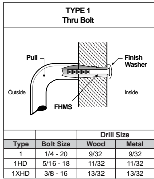
Wood or Metal Door - Type 1
