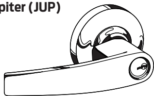
Jupiter (JUP)
