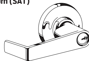
Saturn (SAT)
