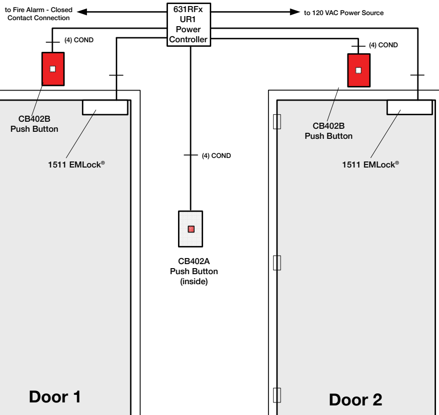
1511 EMLock®
